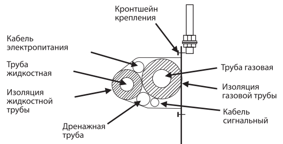
Рисунок 34 - Схема связывания трассы
