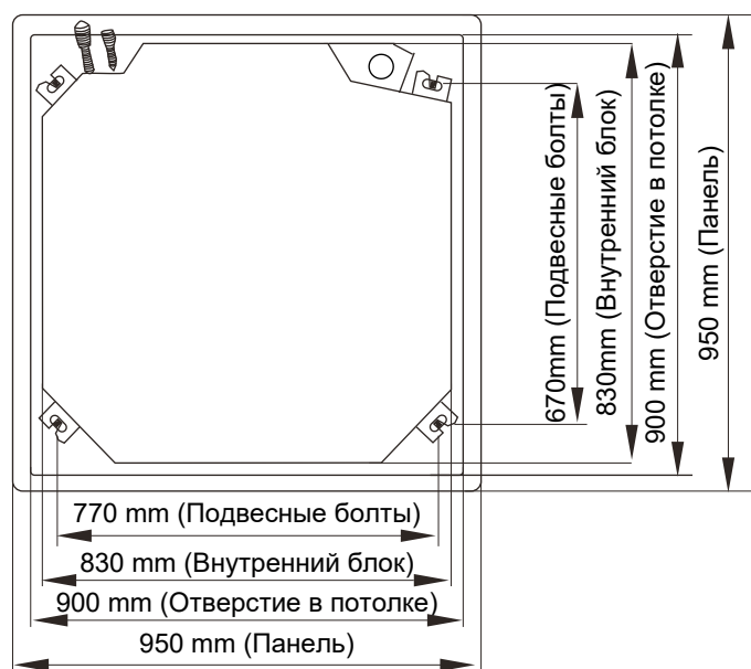
Рисунок 14 - Монтажные размеры внутренних блоков кассетного типа
