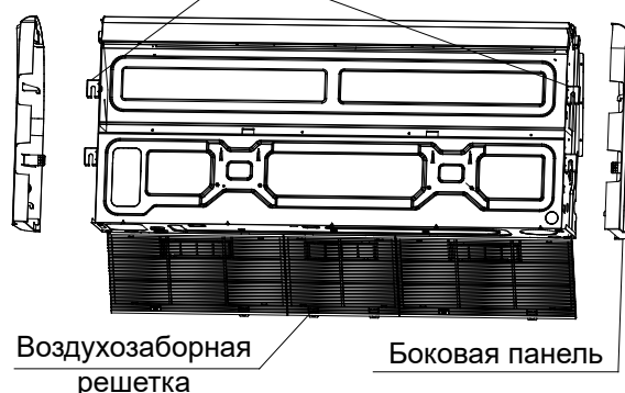
Рисунок 27 - Подготовка к монтажу внутреннего блока напольно-потолочного типа
