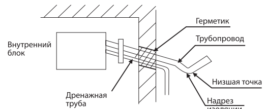
Рисунок 35 - Схема изгиба трубопроводов
