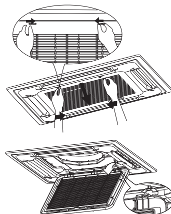
Рисунок 11 - Снятие воздухозаборной решетки внутренних блоков кассетного типа
