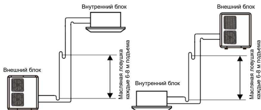
Рисунок 32 - Схема выполнения масляных ловушек
