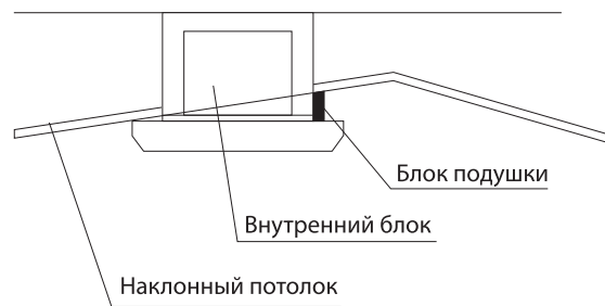
Рисунок 16 - Установка внутреннего блока на наклонном потолке
