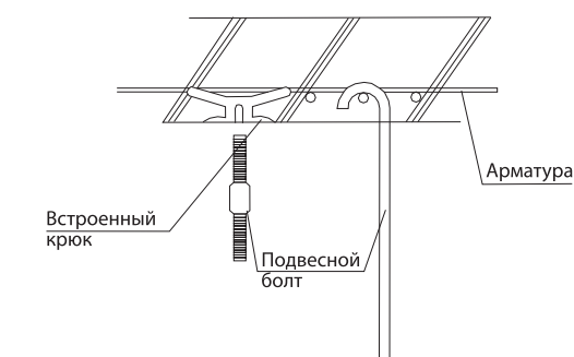
Рисунок 24 - Крепление подвесных болтов к основанию
