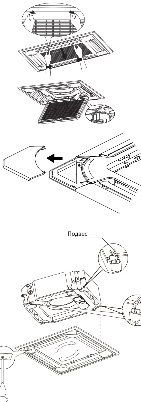
Рисунок 21 - Установка панели внутреннего блока
