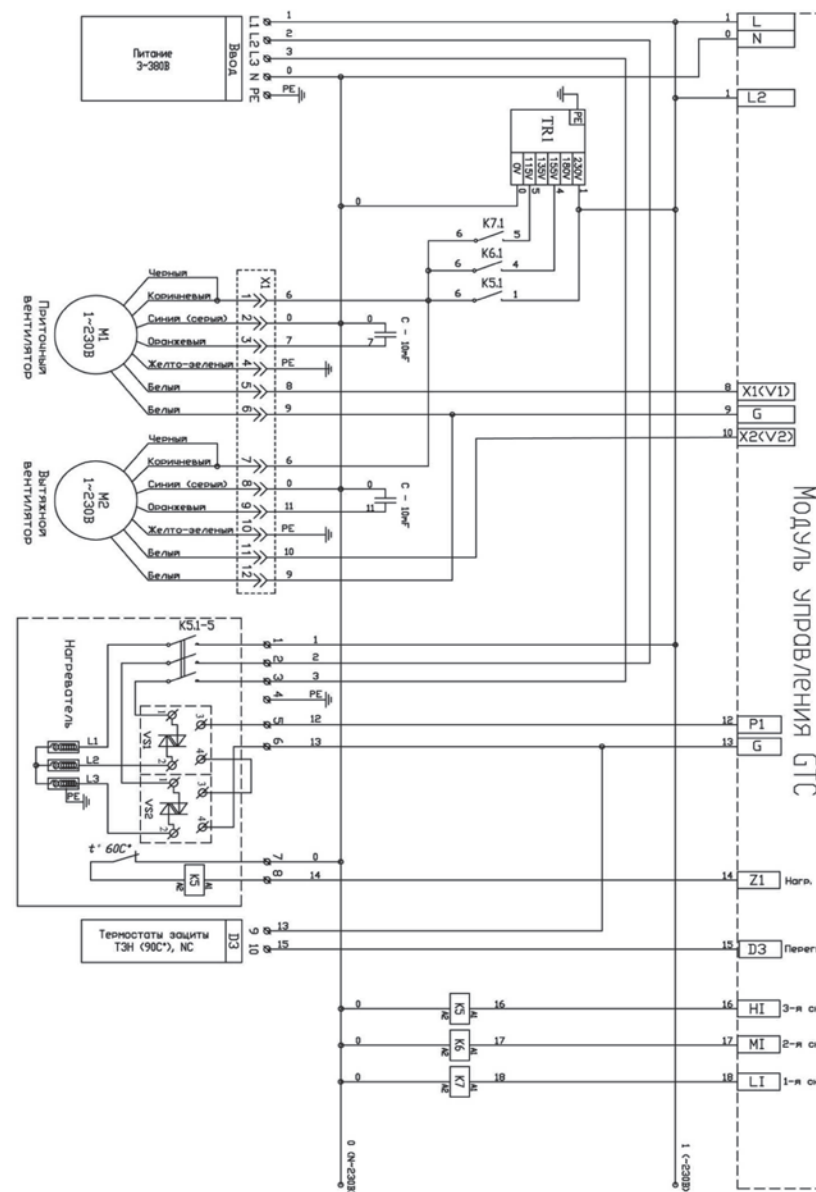
Схема ZPVP 2000 HE
