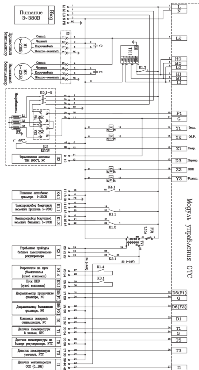
Схема ZPVP 1000 HE, ZPVP 1500 HE
