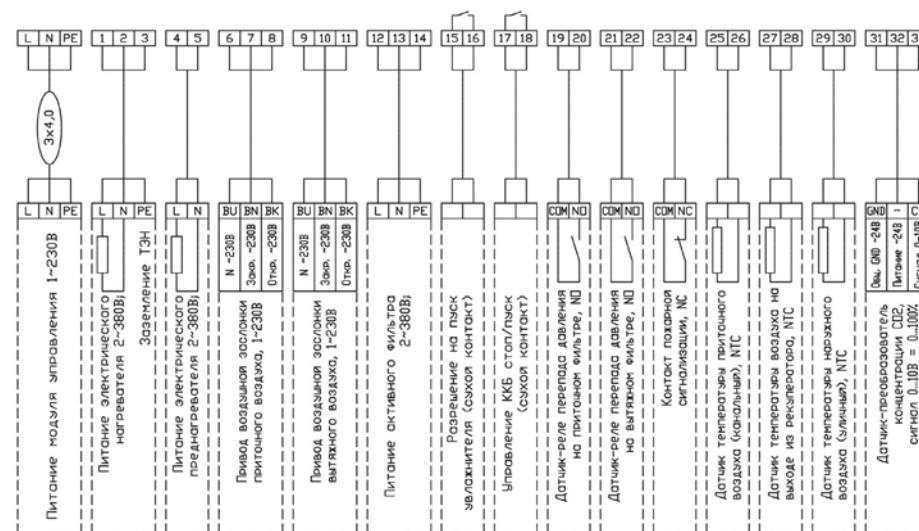
Схема подключения ZPVP 450 PE, ZPVP 800 PE
