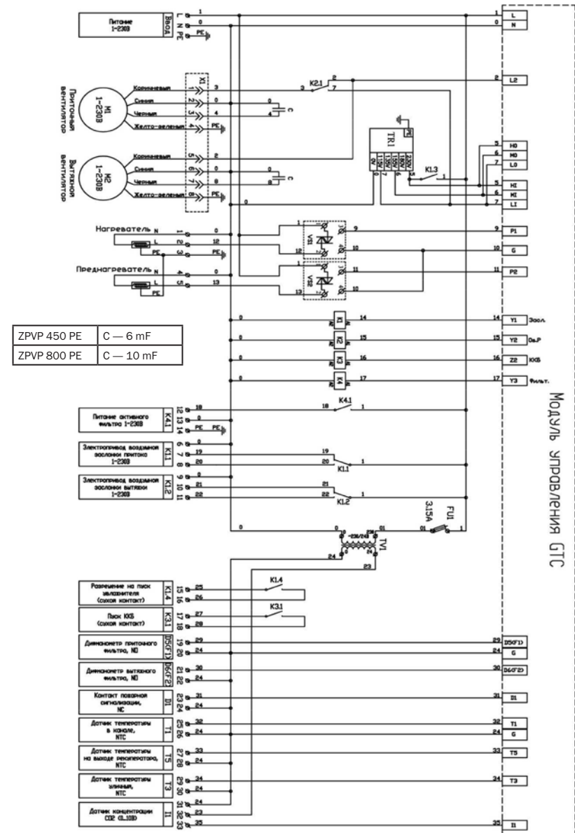
Схема автоматики ZPVP 450 PE, ZPVP 800 PE
