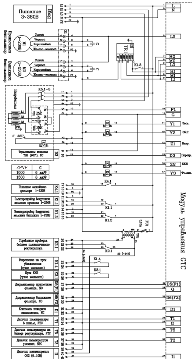
Схема автоматики ZPVP 1000 PE, ZPVP 1500 PE
