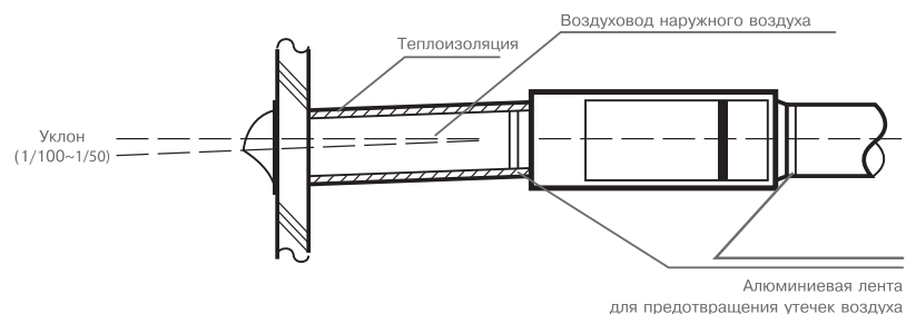
Схема монтажа системы
