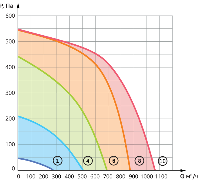
На графике указаны границы производительности установки и скорости для автоматики GTC.
