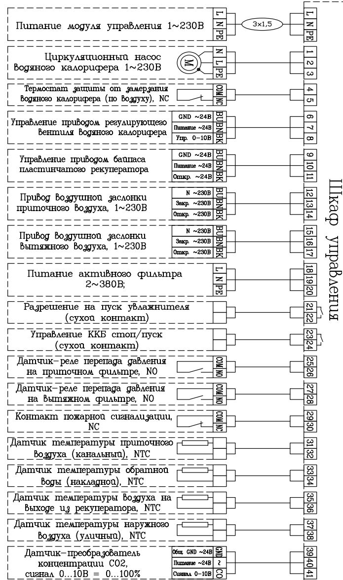
Схема ZPVP 1000 PW, ZPVP 1500 PW
