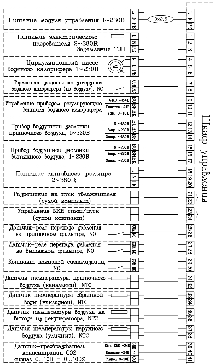
Схема ZPVP 450 VW, ZPVP 800 VW
