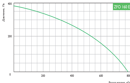
Условия испытаний 505 м³/ч, 200 Па
