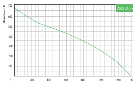
Условия испытаний 600 м³/ч, 243 Па
