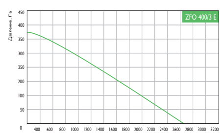
Условия испытаний 1800 м³/ч, 140 Па
