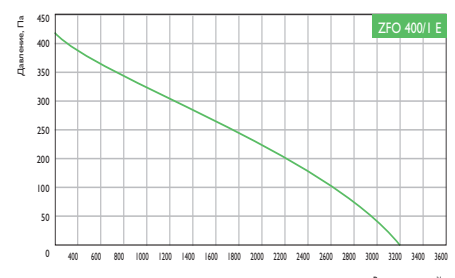
Условия испытаний 2200 м³/ч, 200 Па
