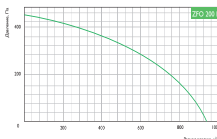
Условия испытаний 610 м³/ч, 195 Па
