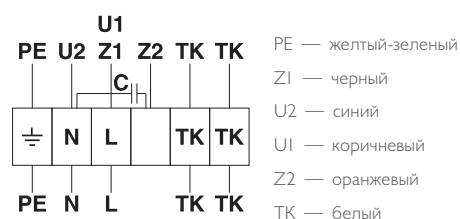
Схема №1 (230 В, 1 фаза)
