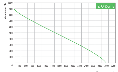
Условия испытаний 2230 м³/ч, 240 Па
