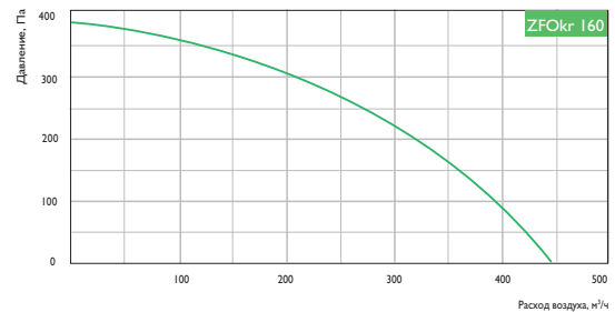
Условия испытаний 300 м³/ч, 220 Па
