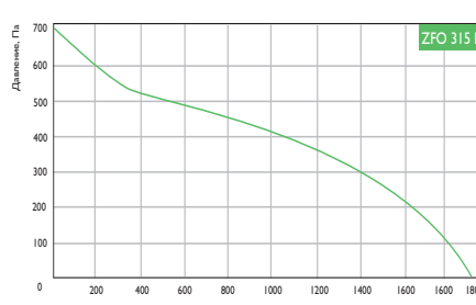
Условия испытаний 1200 м³/ч, 195 Па
